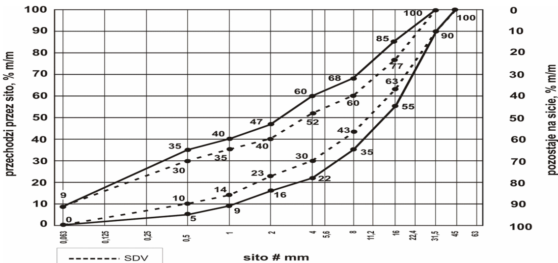
Rys. 1. Uziarnienie mieszanki niezwiązanej 0/31,5 dla warstwy nawierzchniowej
